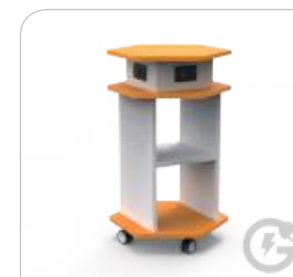
Modulo centrale alimentato con 4 prese Schuko + 8 USB Module Central N°4 220V. + N°8 USB
